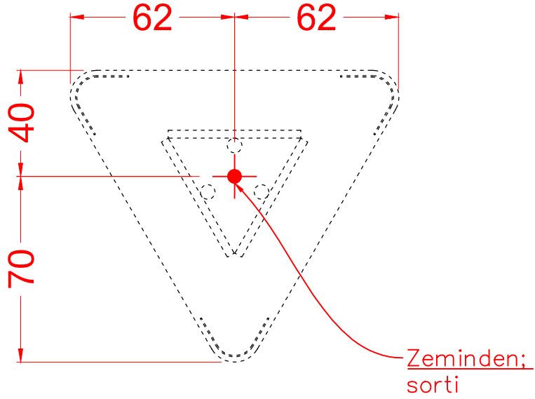
ÜST GÖRÜNÜŞ
